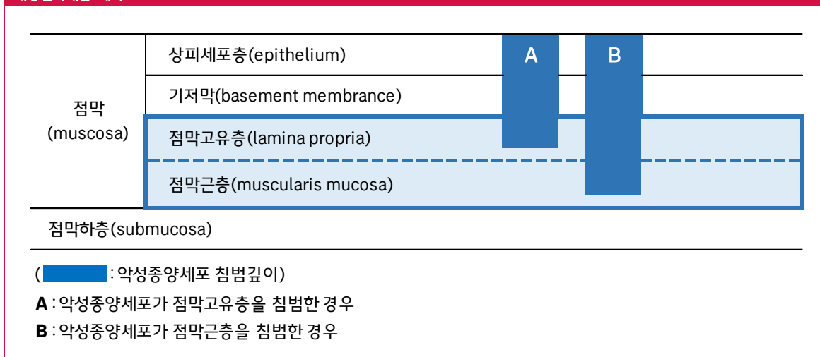
대장점막내암 예시
